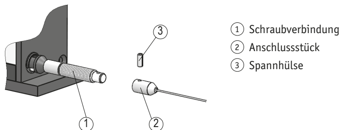
Abb. 9: Seilverlängerung
