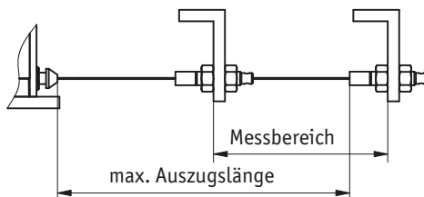
Abb. 2: Prüfung Auszugslänge
