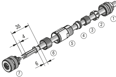
Abb. 10: Gegenstecker M12 gerade
