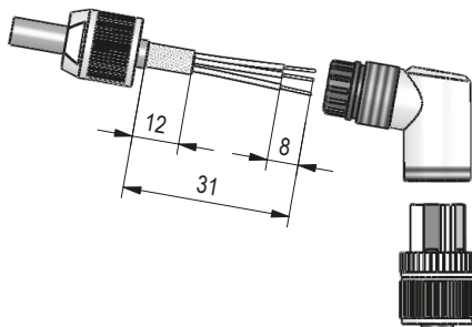
Abb. 11: Gegenstecker M12 gewinkelt
