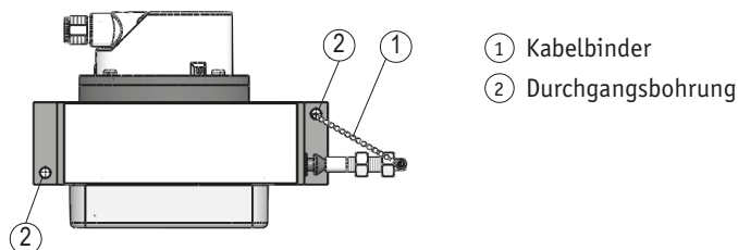
Abb. 3: Montage
