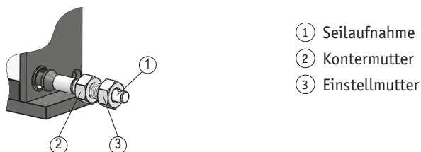
Abb. 4: Seilaufnahme mit Gewinde
