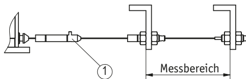
Abb. 8: Messbereich Seilverlängerung
