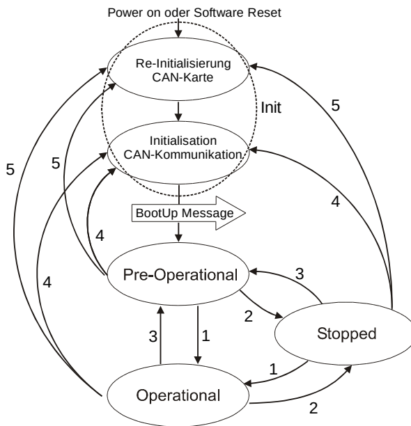
Abb. 1: CAN-Zustands-Diagramm
