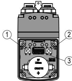
Abb. 13: Bedienelemente
