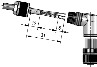
Abb. 16: Gegenstecker M12 gewinkelt
