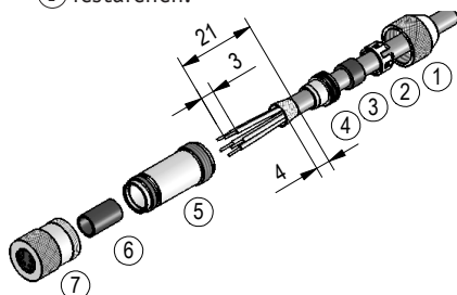
Abb. 15: Gegenstecker M12 gerade
