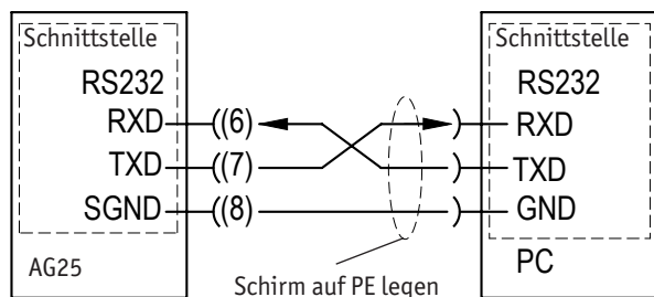
Abb. 10: Anschlussschema Schnittstelle RS232
