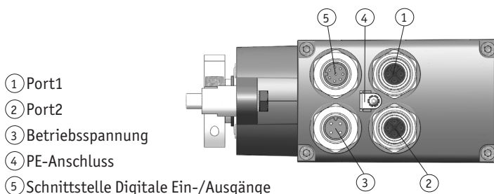
Abb. 7: Anschlussbelegung
