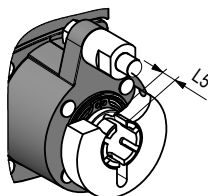
Abb. 6: Klemmring, Welle mit Passfedernut
