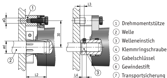
Abb. 1: Einbaumaße
