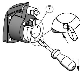
Abb. 5: Transportsicherung
