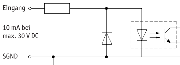
Abb. 9: Eingangsschaltung
