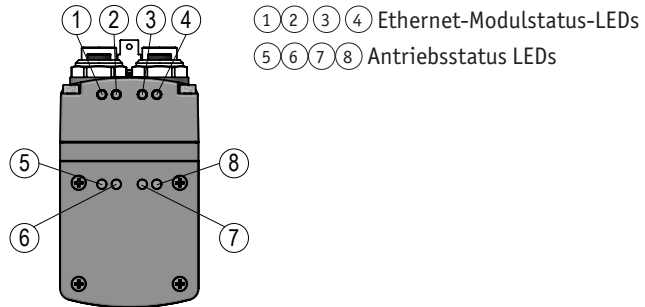
Abb. 12: Statusanzeige
