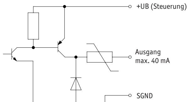
Abb. 8: Ausgangsschaltung
